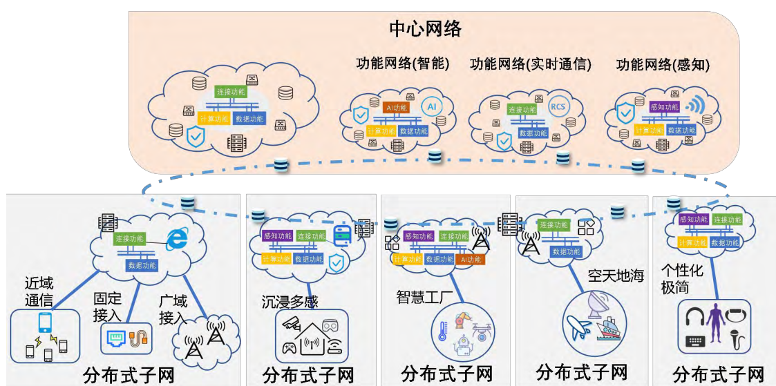
图 3-1 6G 分布式组网形态
