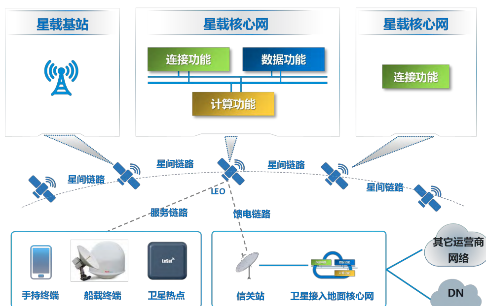
图 2-3 星载核心网典型组网架构
